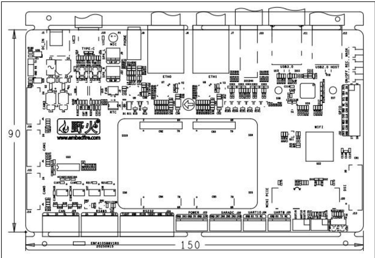
图 5.2-1 鲁班猫 3BTB 底板正面机械尺寸图
