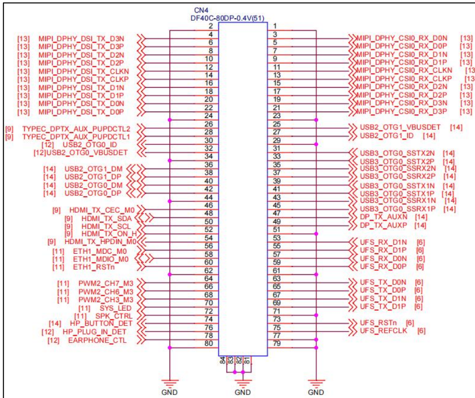
图 4.6-4 CN4 连接器原理图
