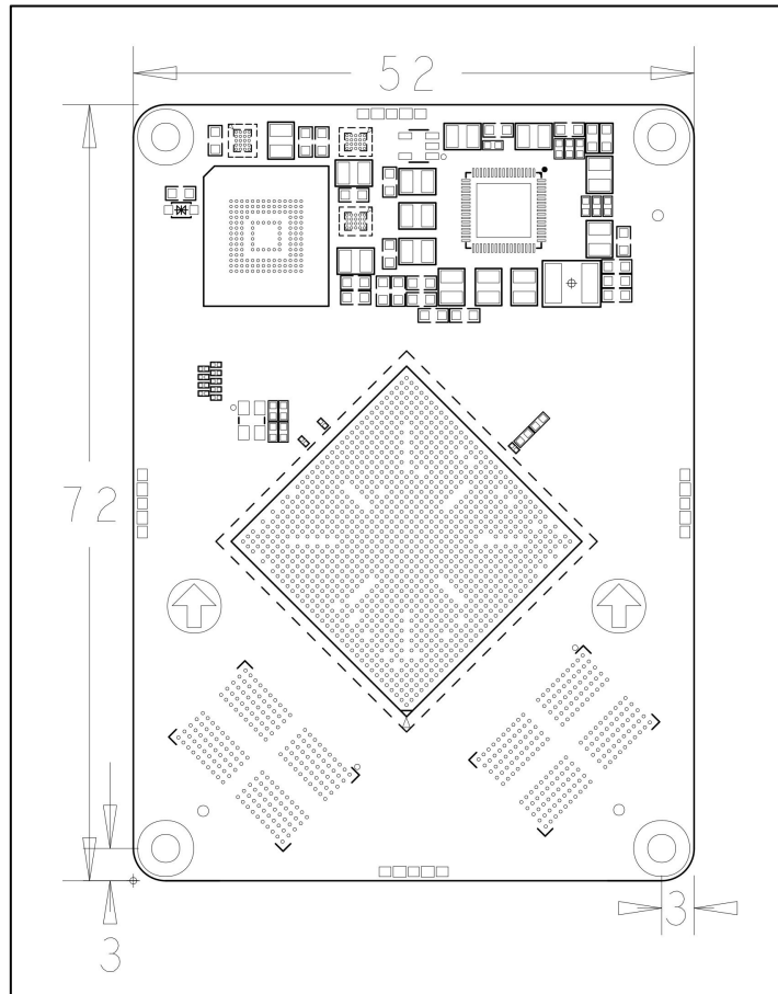
图 4.2-1 鲁班猫 3BTB 核心板正面机械尺寸图
