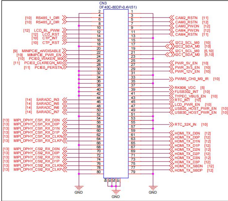
图 4.6-3 CN3 连接原理图
