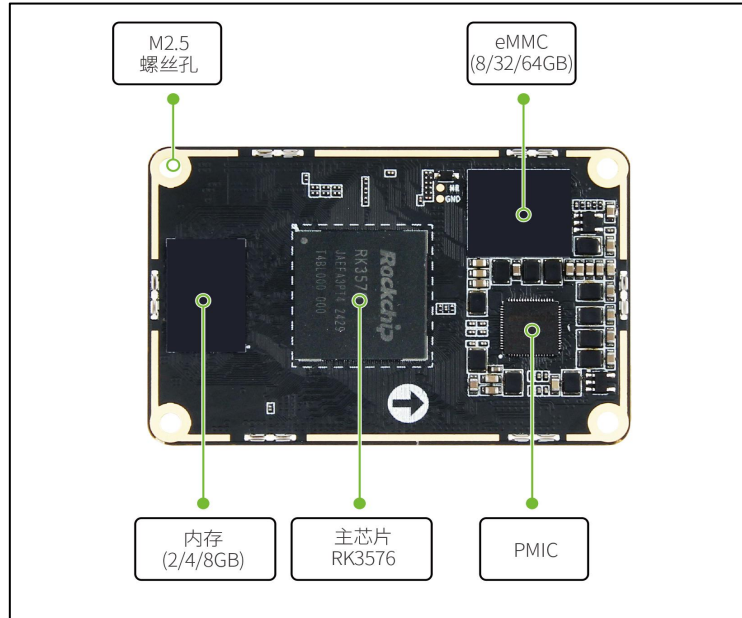
图 4.1-1 鲁班猫 3BTB 核心板正面视图
